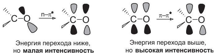
Рис. 32. Запрещенный ( n \rightarrow \pi^* ) и разрешенный ( \pi \rightarrow \pi^* ) по симметрии электронные переходы в карбонильной группе
