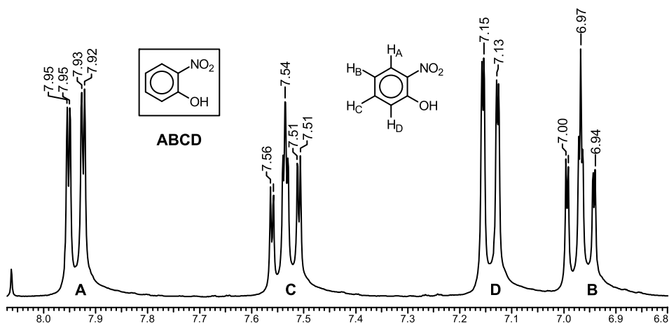
Рис. 73. Спектр ЯМР ^1H 2-нитрофенола
