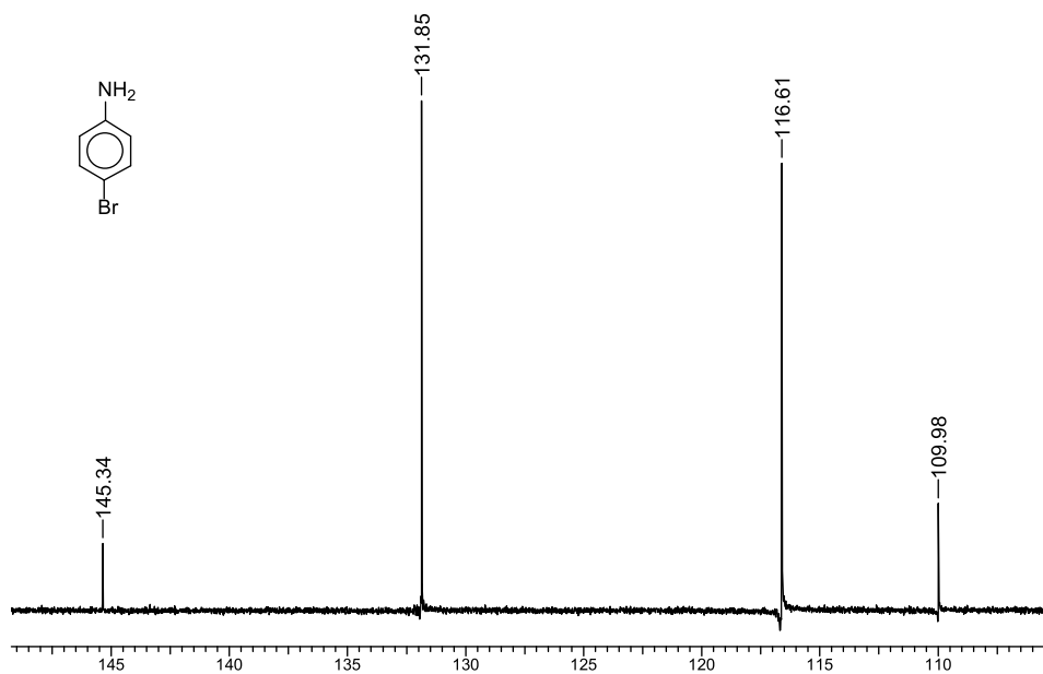
В7.2.6. Спектры ЯМР ^1\text{H} и ^{13}\text{C} 4-броманилина
