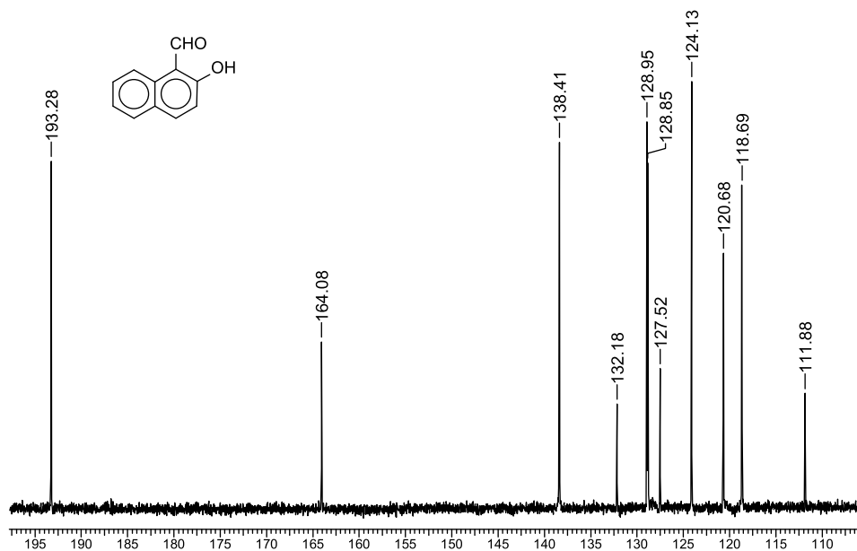
Б7.7.1. Спектры ЯМР 1 H и 13 C 2-гидрокси-1-нафальдегида
