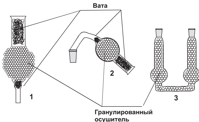
Рис. 9. Осушительные трубки: 1 – хлоркальцевая трубка с одним шаром, используемая при перегонке с прямым холодильником; 2 – хлоркальцевая трубка с одним шаром и шлифованным керном, устанавливаемая на выходе обратного холодильника; 3 – U-образная трубка (обычно используется для осушки потока газа)
