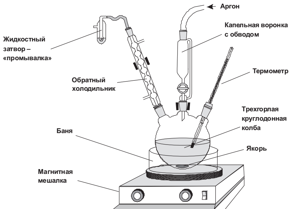
Рис. 14. Прибор для проведения синтеза в инертной атмосфере при охлаждении с контролем температуры
