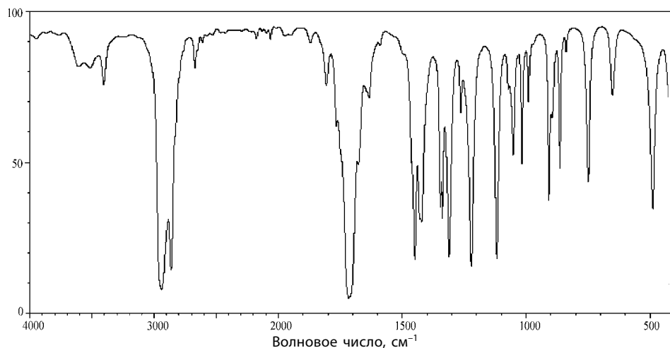
Рис. 30. ИК-Спектр циклогексанола
